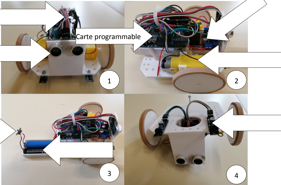
Document n°1 : les composants mécatronique du robot.
